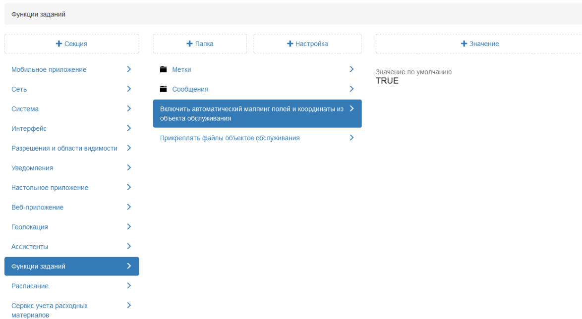
Рис. 2.318: Автоматический маппинг полей и координаты из объекта обслуживания
