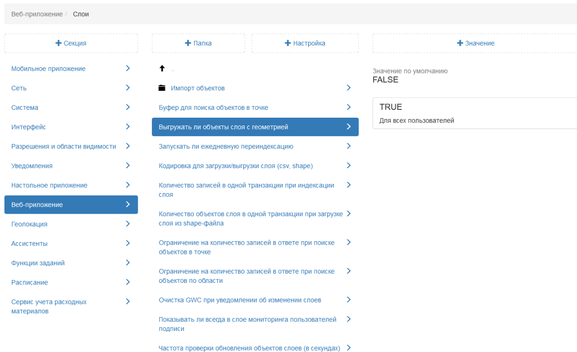
Рис. 2.255: Настройка выгрузки слоя с геометрией объектов
