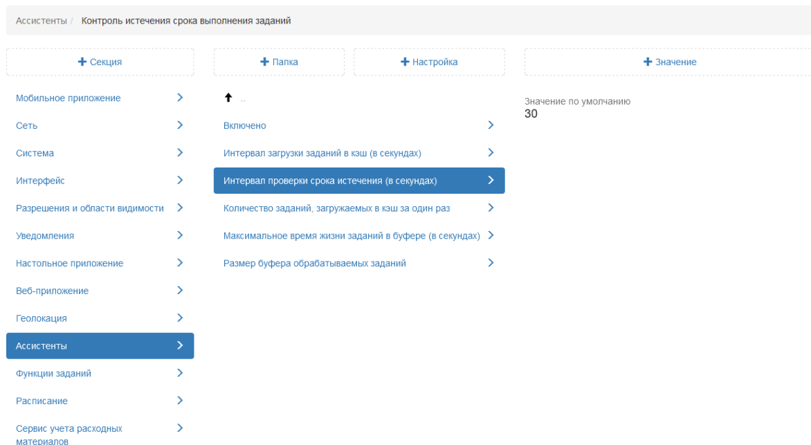
Рис. 2.303: Интервал проверки истечения срока
