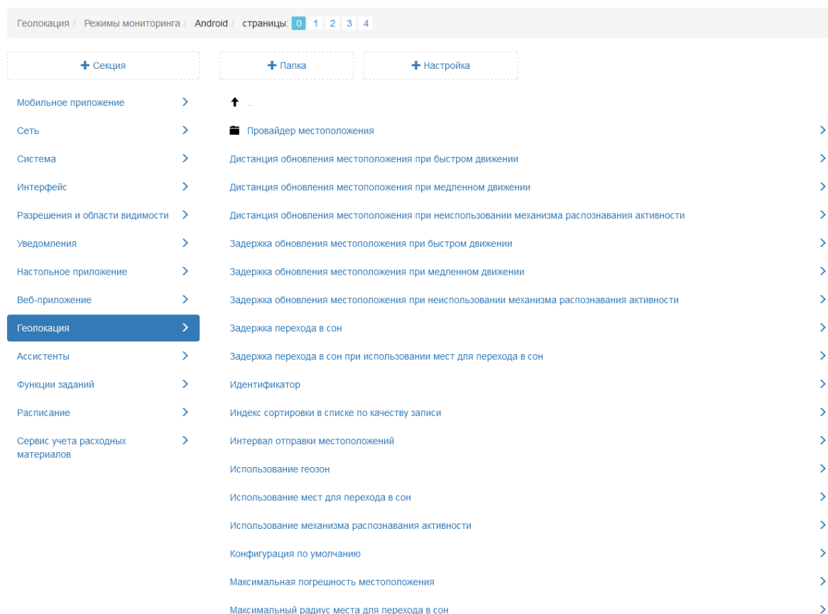
Рис. 2.270: Настройки режима мониторинга для операционной системы Android
