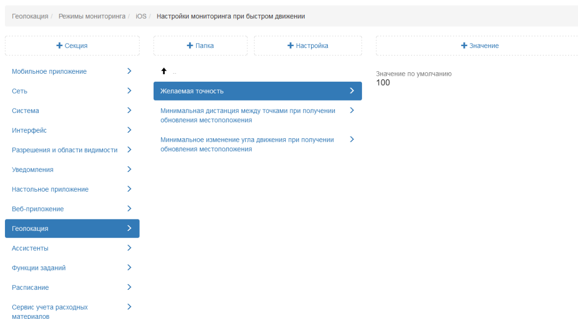
Рис. 2.275: Желаемая точность при медленном движении
