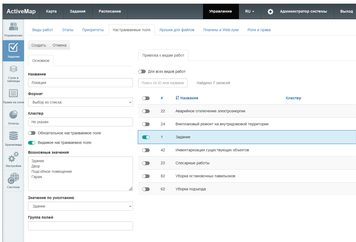
Рис. 2.79: Создание настраиваемого поля, вкладки «Основное» и «Привязка к видам работ»
