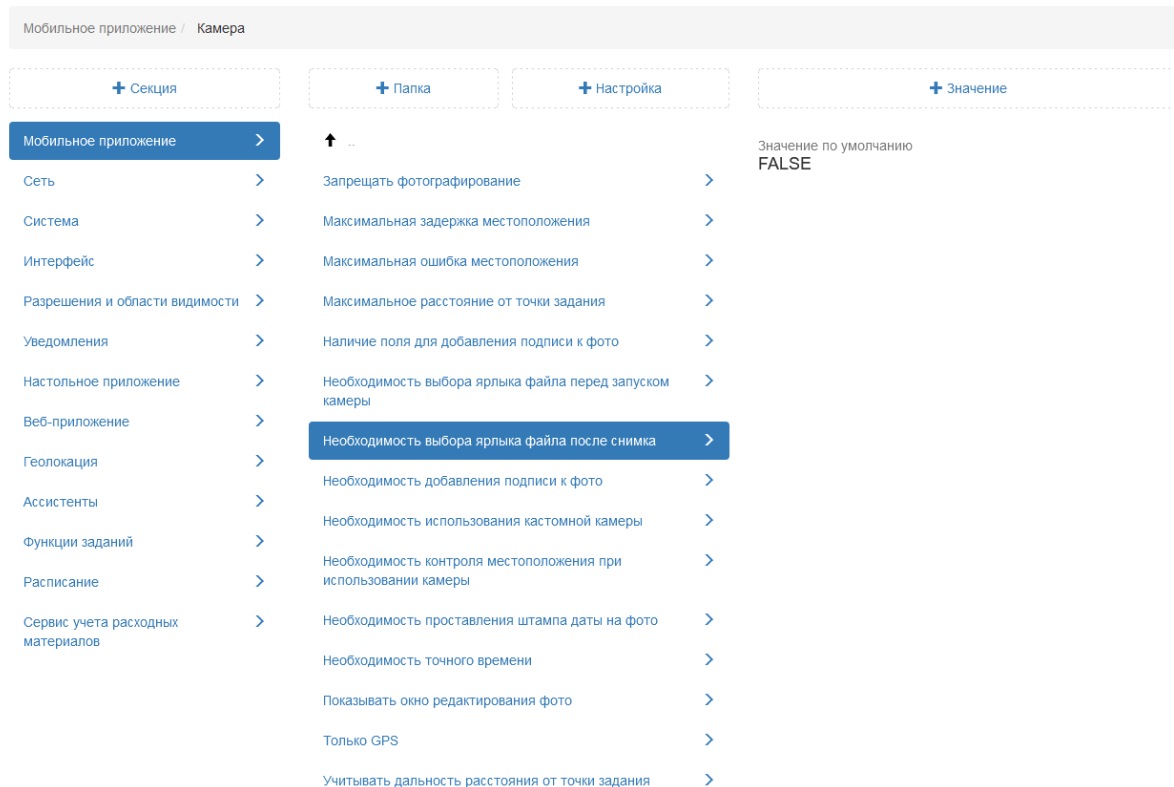
Рис. 2.155: Выбор ярлыка файла после запуска камеры
