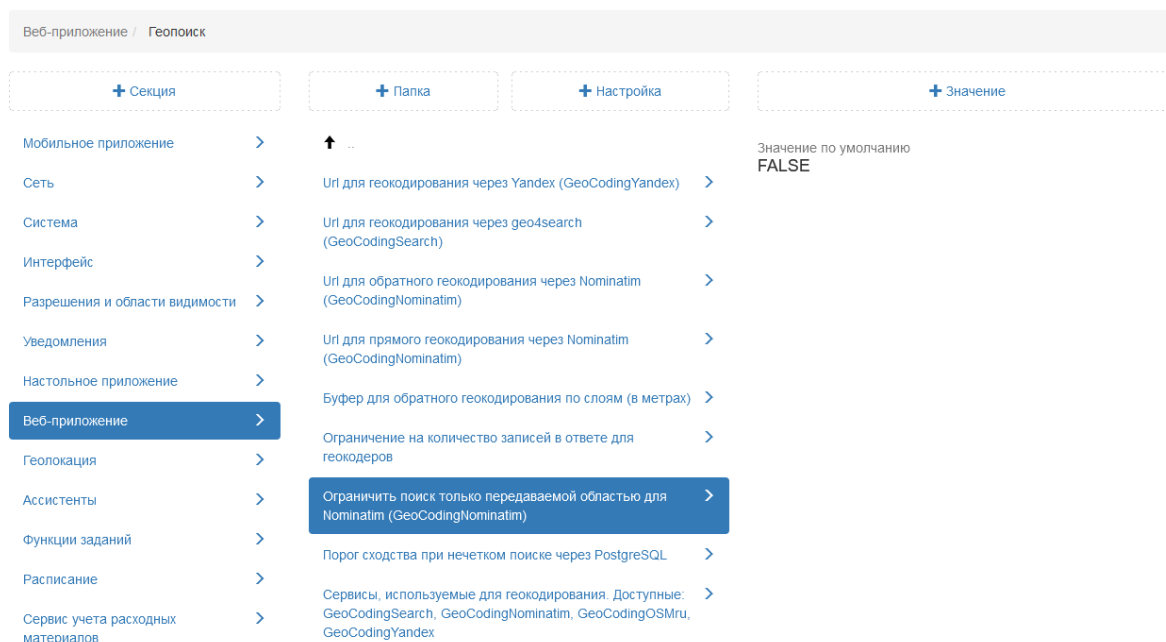
Рис. 2.238: Ограничение поиска только передаваемой областью для Nominatim
