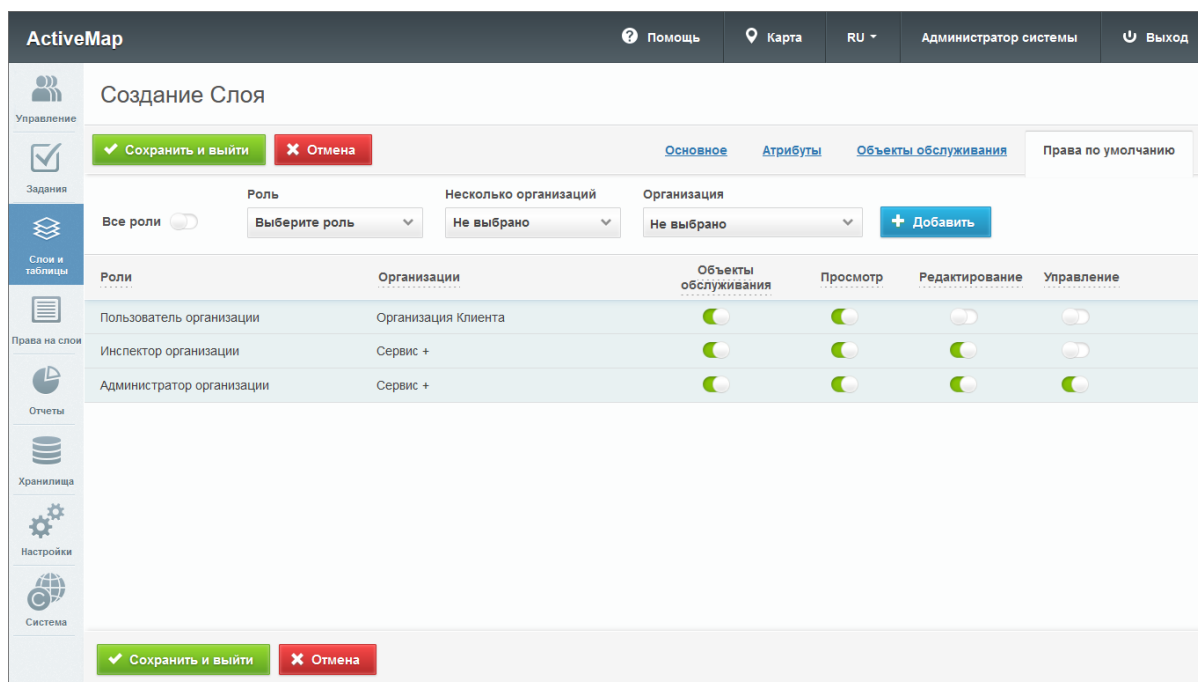
Рис. 2.100: Вкладка «Права по умолчанию»
