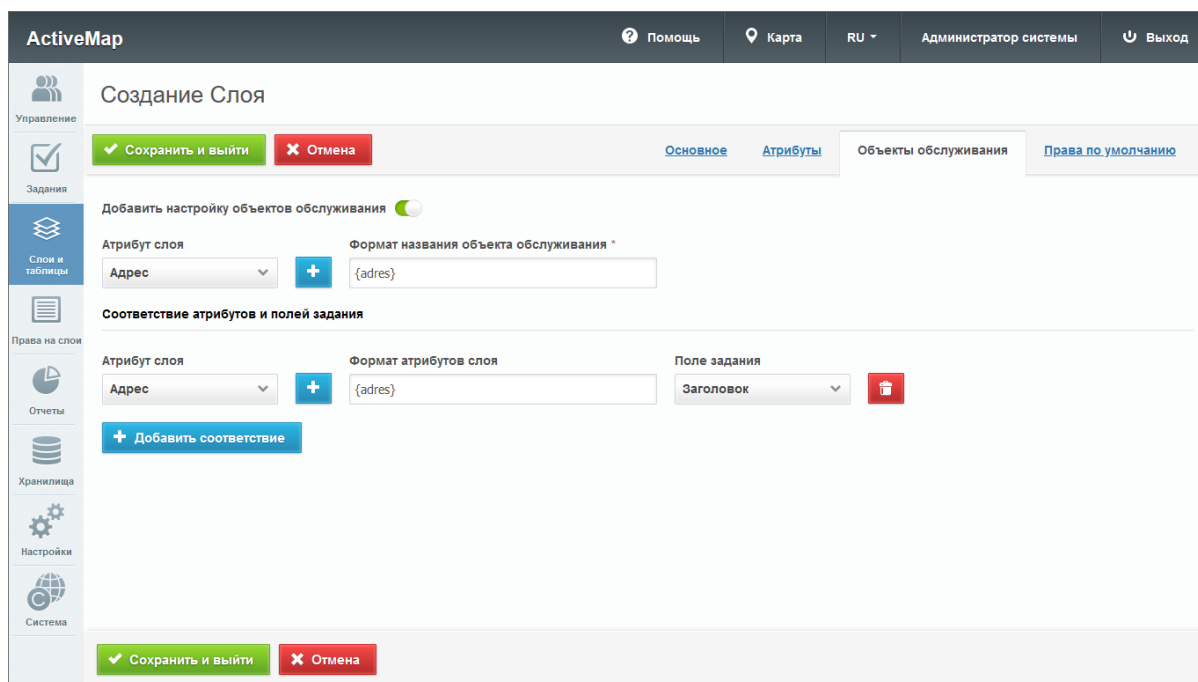
Рис. 2.99: Вкладка «Объекты обслуживания»
