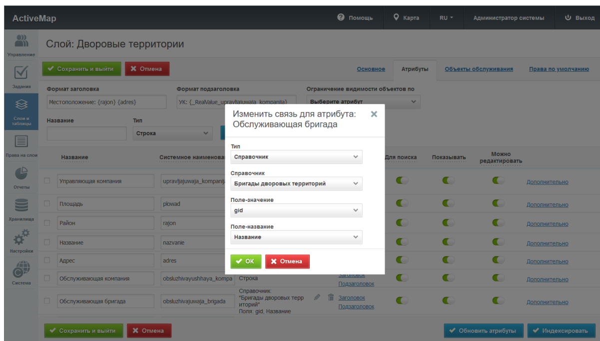
Рис. 2.108: Изменение связи для атрибута
