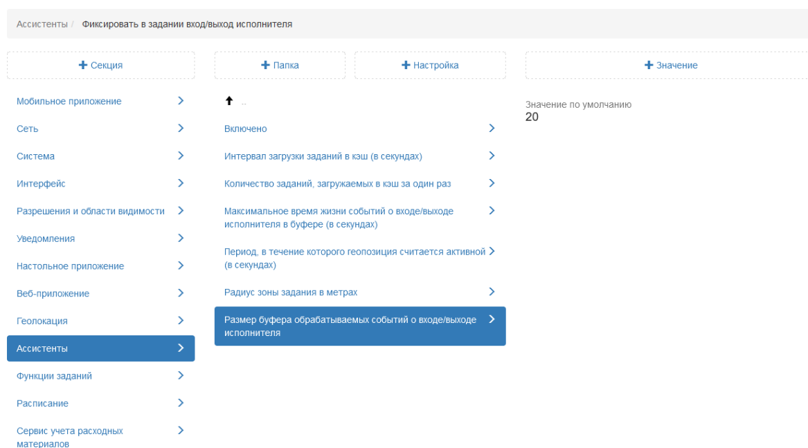
Рис. 2.310: Размер буфера обрабатываемых событий о входе/выходе исполнителя
