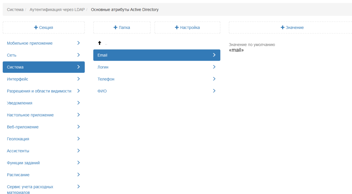
Рис. 2.199: Основные атрибуты Active Directory
