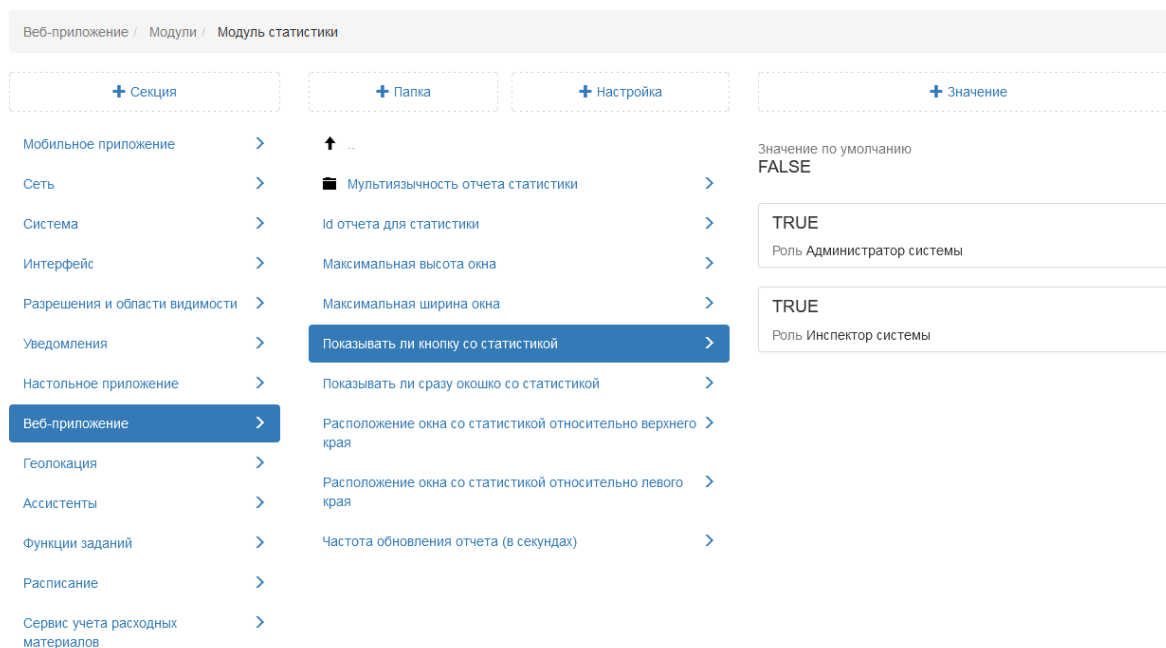
Рис. 2.243: Показывать ли кнопку со статистикой
