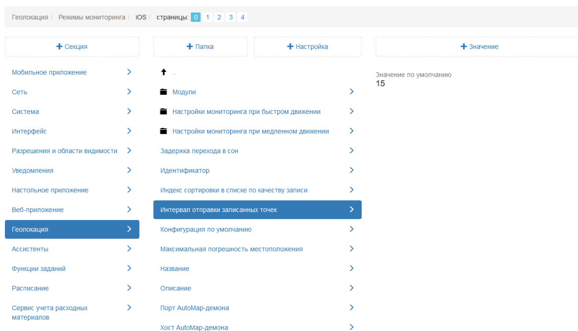
Рис. 2.284: Интервал отправки записанных точек
