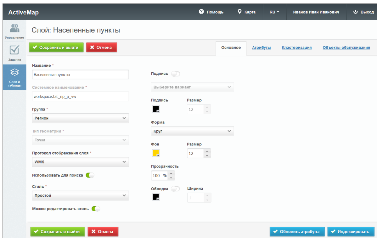
Рис. 2.99: Редактирование информации о слое
